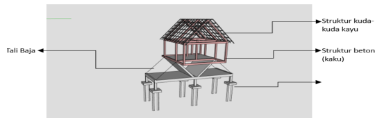
Gambar 18. Struktur Bangunan Penginapan
