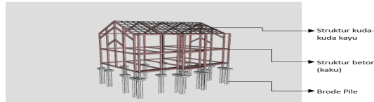
Gambar 17. Struktur Bangunan Indoor Wedding
