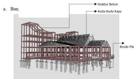
Gambar 15. Struktur Bangunan Utama
