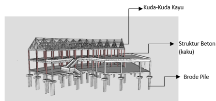
Gambar 16. Struktur Bangunan Suvernir
